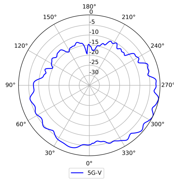
5G (Vertical)
