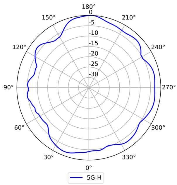
5G (Horizontal)
