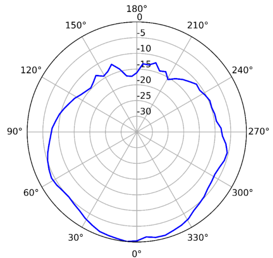
5GHz (Vertical)
