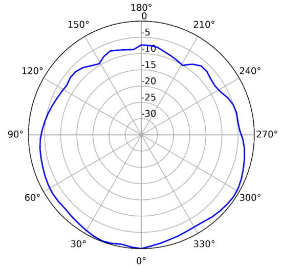
2.4GHz (Vertical)
