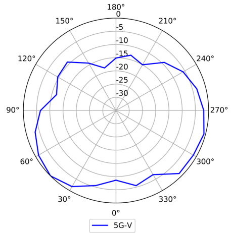
5G (Vertical)
