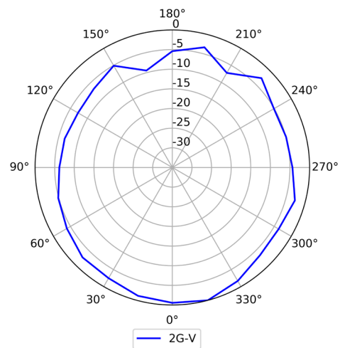
2.4G (Vertical)
