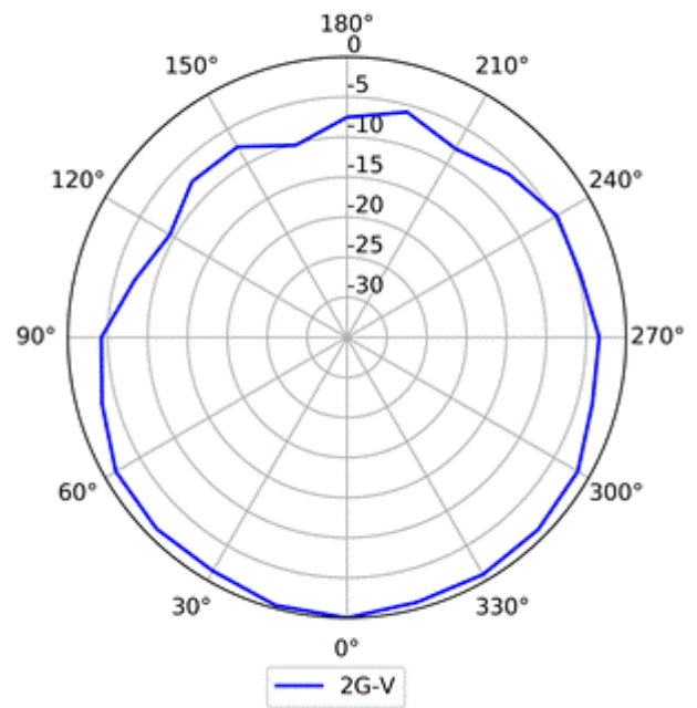
2.4G (Vertical)
