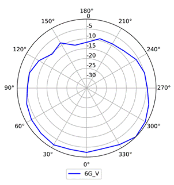
6G (Vertical)
