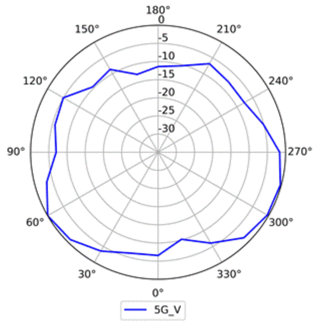
5G (Vertical)
