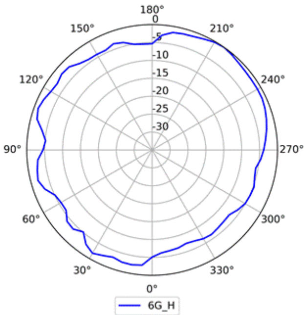
6G (Horizontal)
